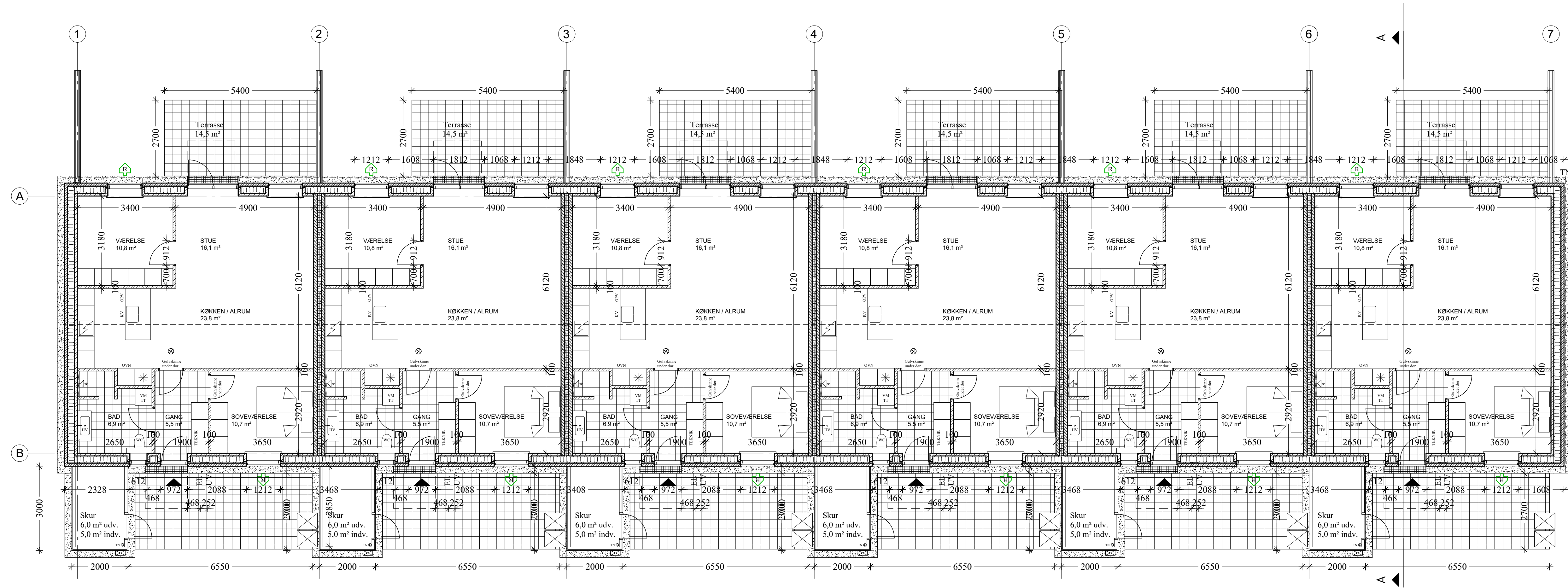
STUEPLAN Rækkehuse, 6 x 90 m 2
